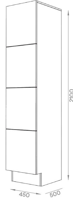
4-Tier 150mm toekick
